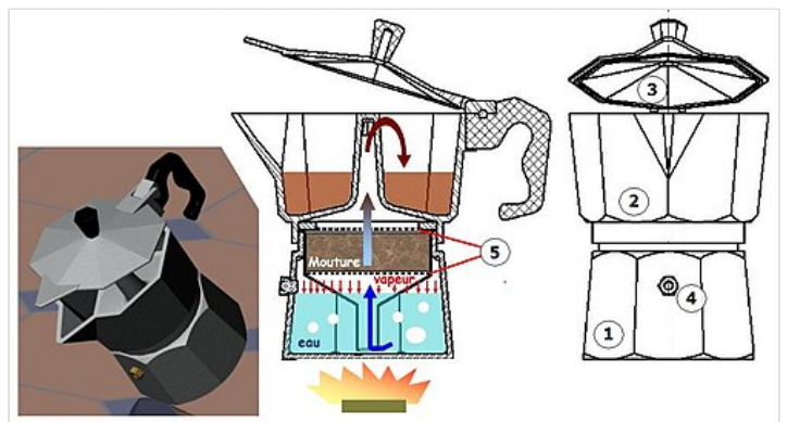
Principe de la cafetière italienne.
